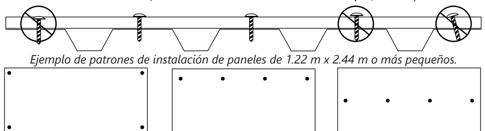
Figura F - Instalación de tornillos ESD
