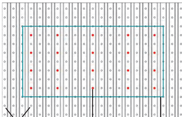
Figura A - Patrón de cuadrícula para estructura acanalada para Invisi-Loc®
